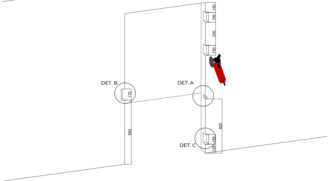
DET. A
